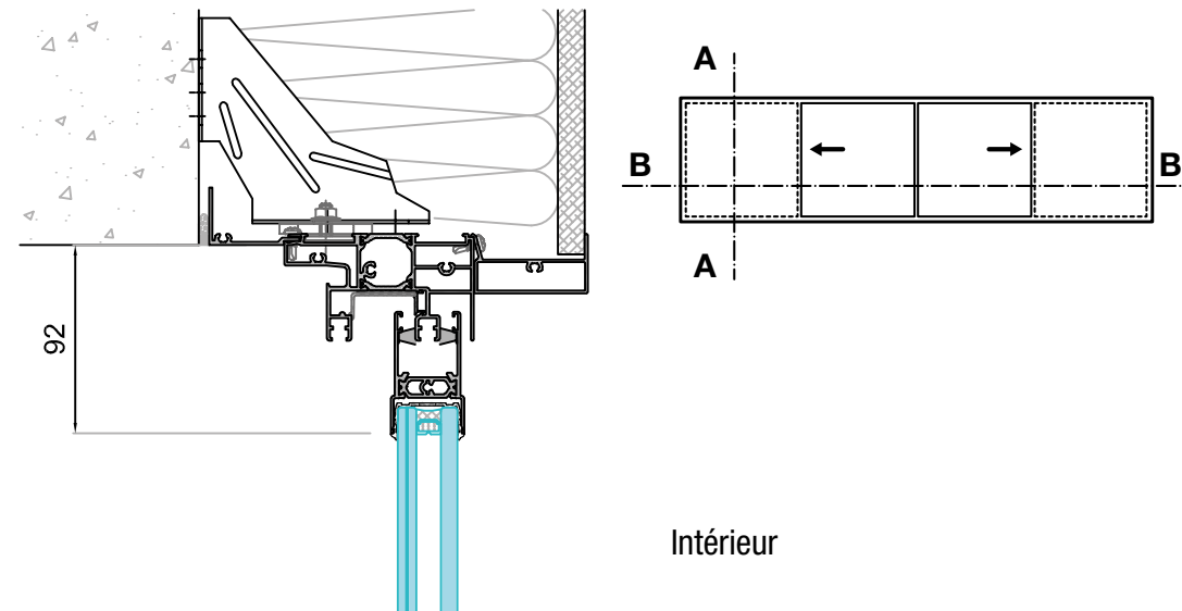
COUPE A-A
