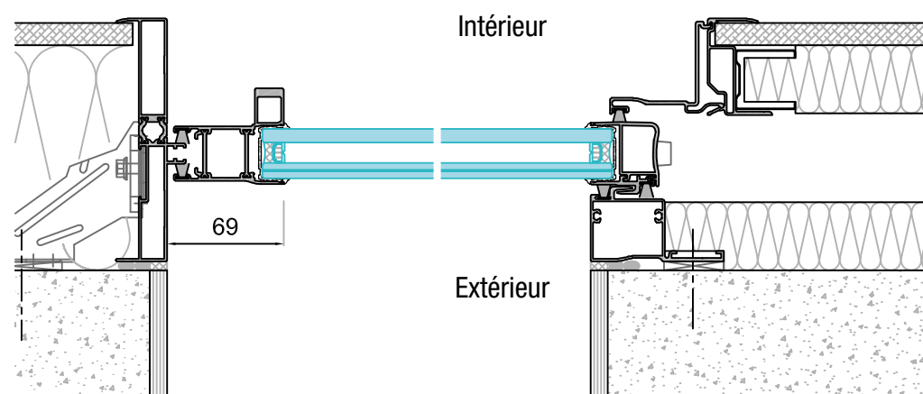
COUPE B-B
