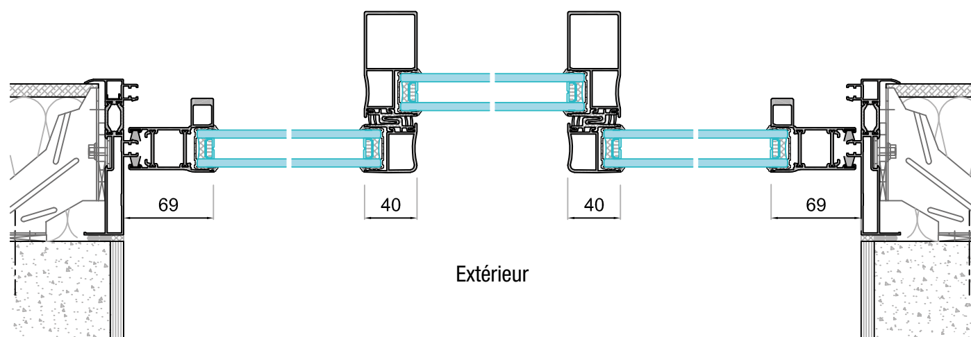
COUPE B-B
