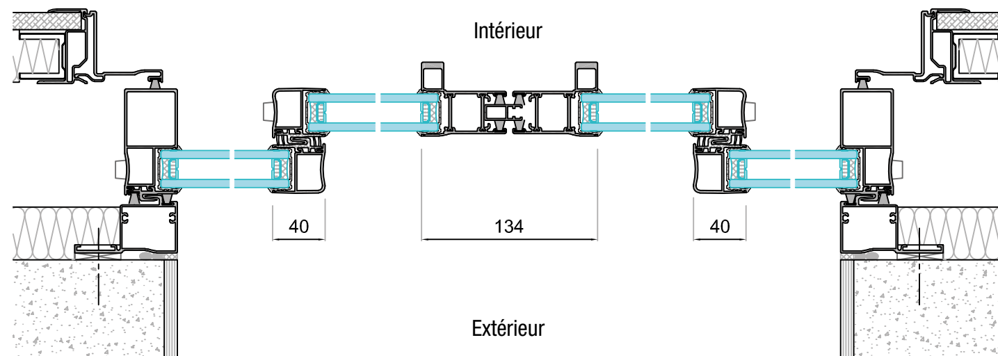
COUPE B-B
