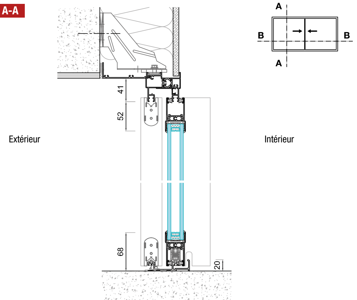
COUPE B-B
