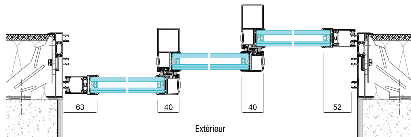
COUPE B-B
