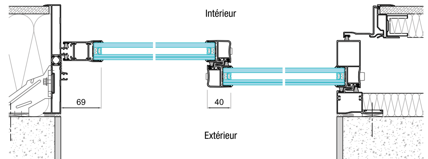
COUPE B-B
