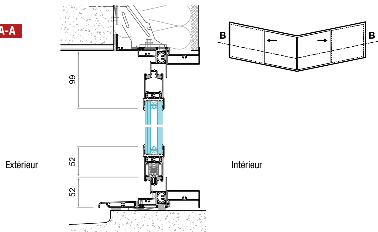
COUPE B-B
