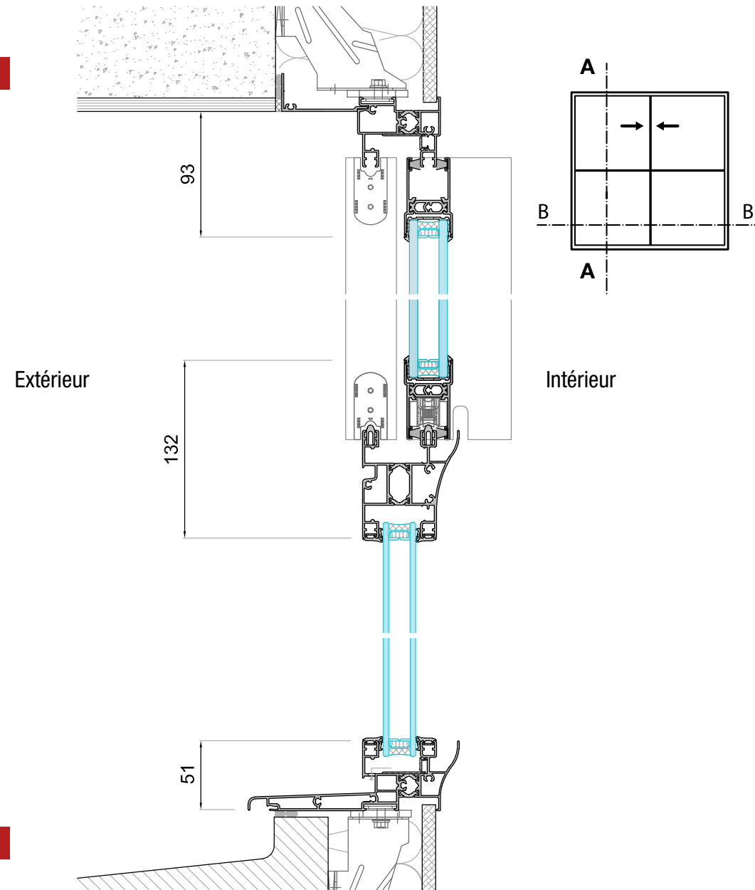
COUPE A-A
