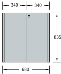
Q 411.31 Door set silver-grey RAL 9006
