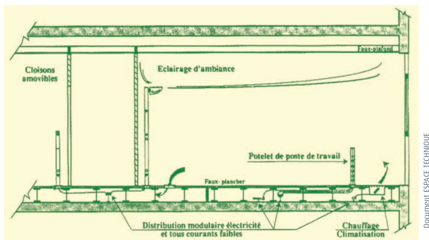
Exemple de conception de bureaux flexibles.
