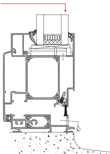
Base 72, ouvrant serrure
