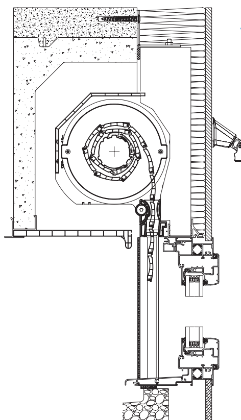
Fenêtre à ouvrant caché et volet bloc-baie demi-linteau
