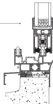
Pose en tableau
