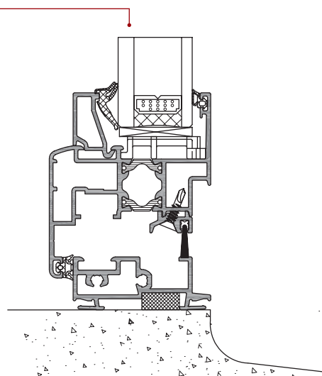
Base 52, ouvrant crémone
