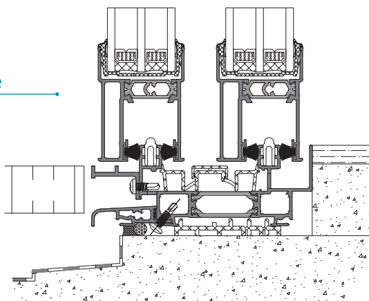
Seuil encastré
