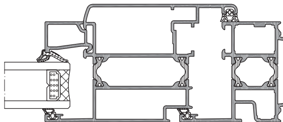
COUPE HORIZONTALE
