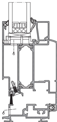
COUPE VERTICALE SEUIL RENFORCÉ
